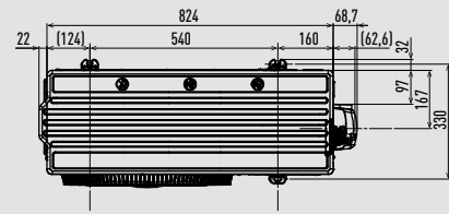
Frontansicht
