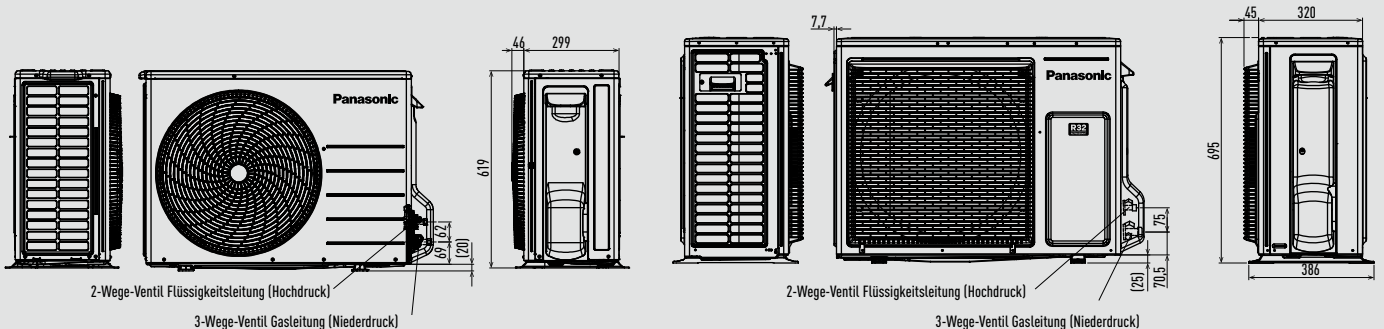
Seitenansicht
