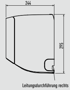
Seitenansicht
