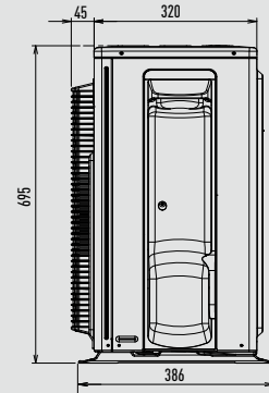
Seitenansicht
