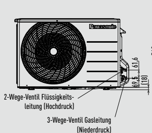
Frontansicht
