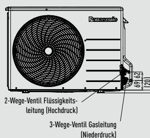
Frontansicht
