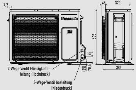
Frontansicht
