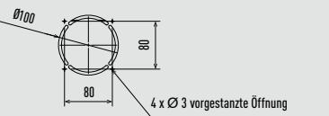
Detailansicht X
