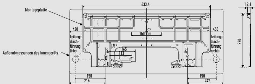
Anordnung von Innengerät und Montageplatte Frontansicht
